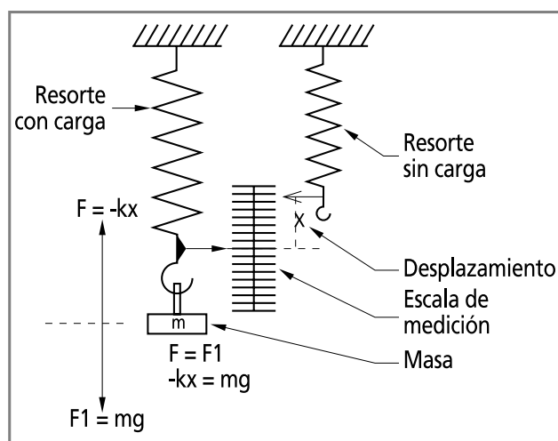
Ilustración 7: Balanza de resorte
