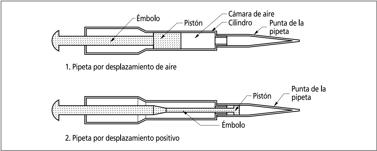
Ilustración 44: Clases de pipetas
