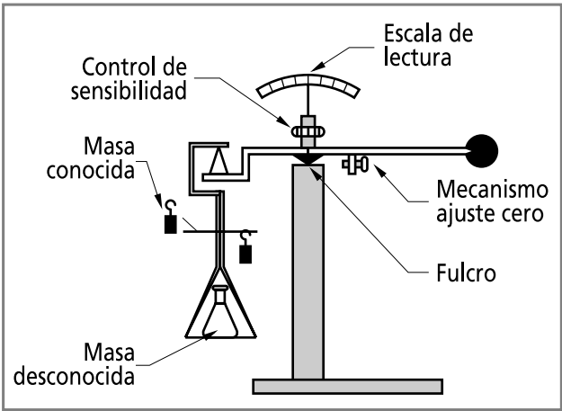
Ilustración 11: Balanza de sustitución
