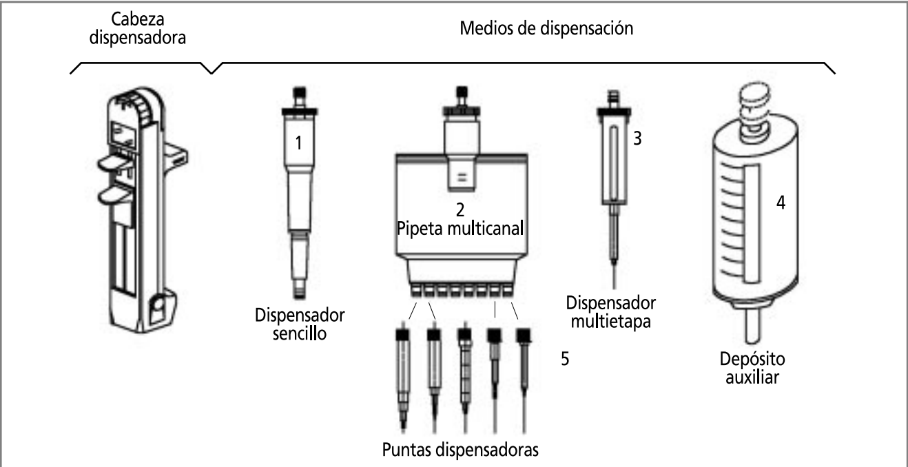
Ilustración 26: Elementos dispensadores
