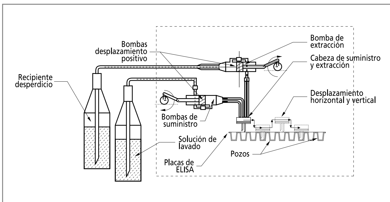
Ilustración 2: Lavador de ELISA
