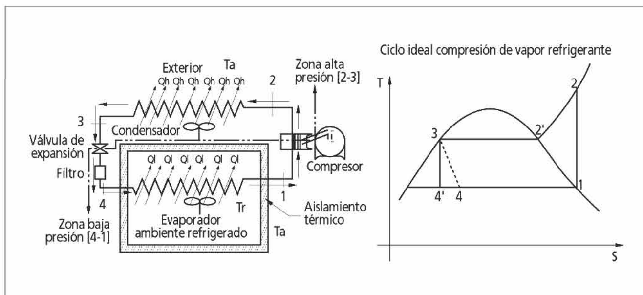
Ilustración 49: Circuito de refrigeración
