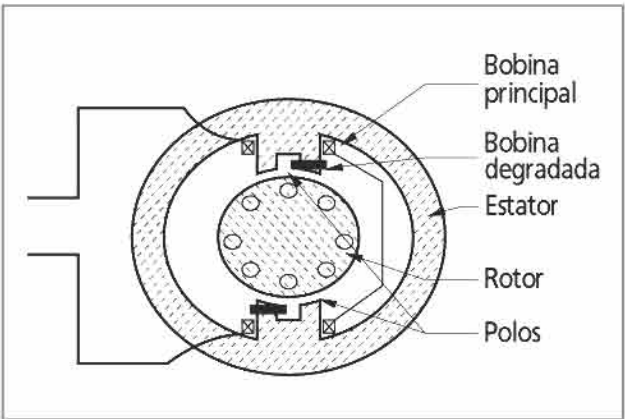
Ilustración 48: Motor de inducción
