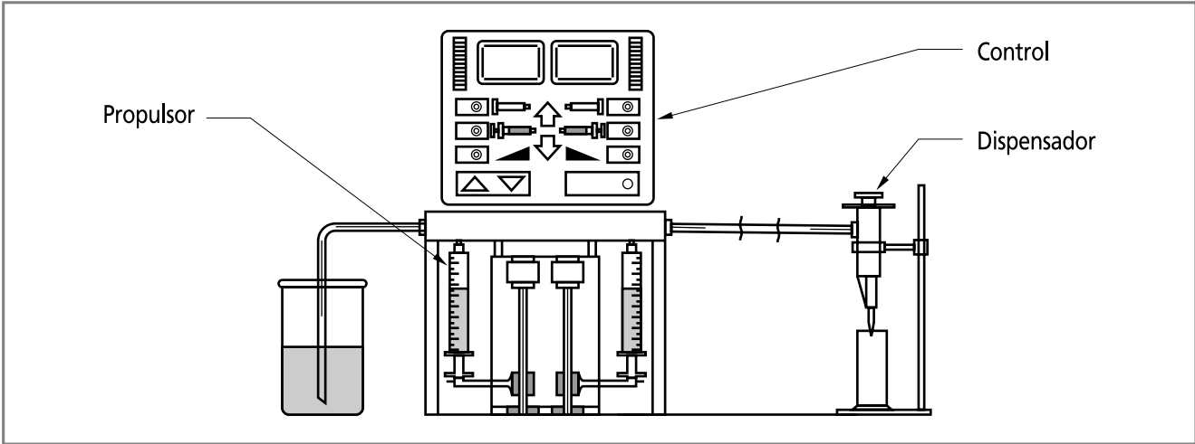
Ilustración 22: Esquema diluidor
