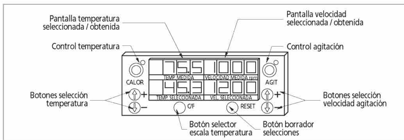
Ilustración 47: Control plato caliente con agitador
