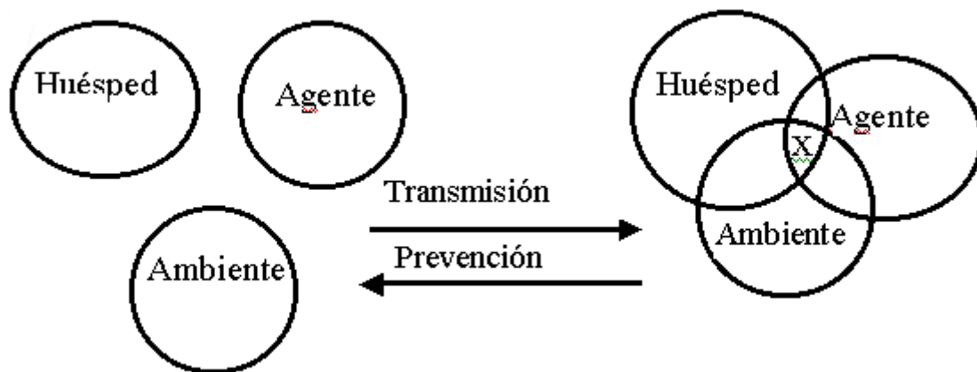
Figura 1: Diagrama ambiente, agente, huésped. Transmisión y prevención.
